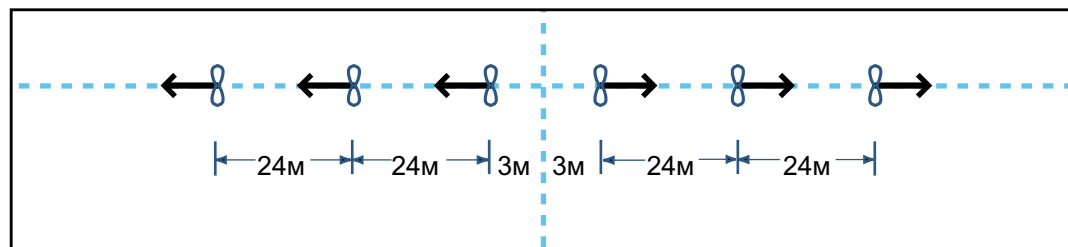
Схема 24: Принцип установки и траектория циркуляции воздуха при использовании лопастных смесителей воздуха в птичнике размером 12м x 52м.
