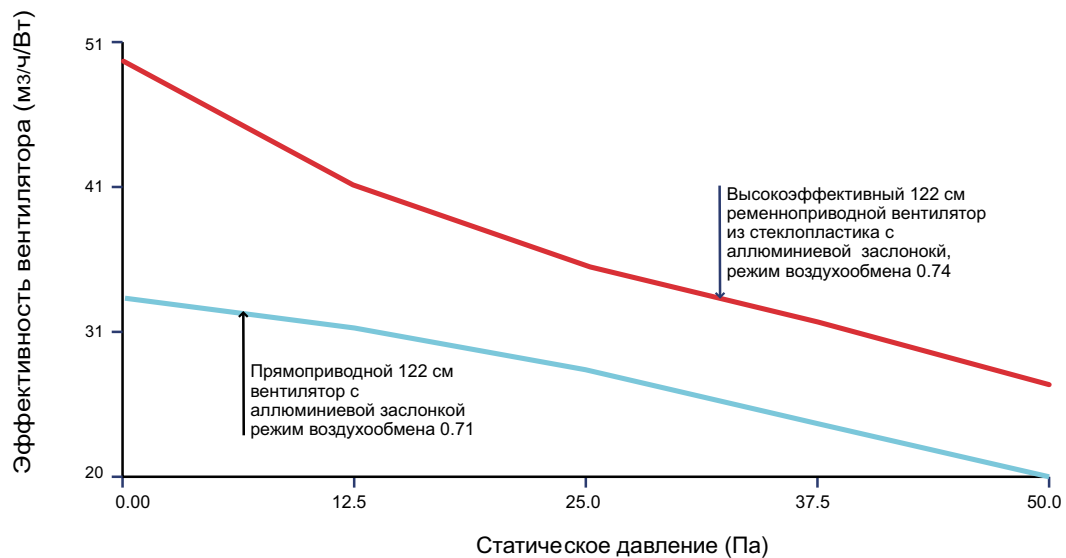
Схема 20: Эффективность вентилятора, выраженная в \text{м}^3/\text{ч}/\text{Вт}
