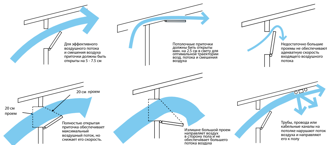
Схема 26: Верное и неверное открытие приточных форточек.
