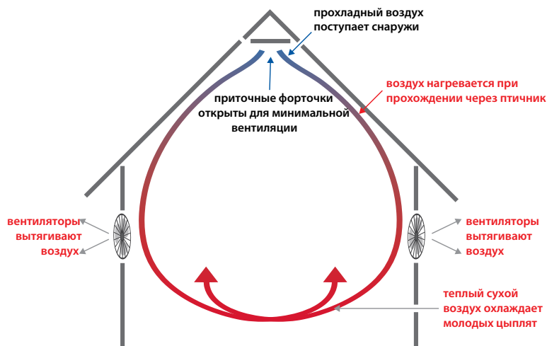
Рис. 6.16: Схема противоточной вентиляции (приточные проемы в крыше)
